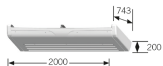
Förångare
