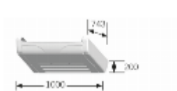
Förångare Medium TMEVX-M Vikt 31kg
