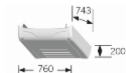
Förångare Small TMEVX-S Vikt 25kg
