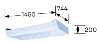
Förångare
